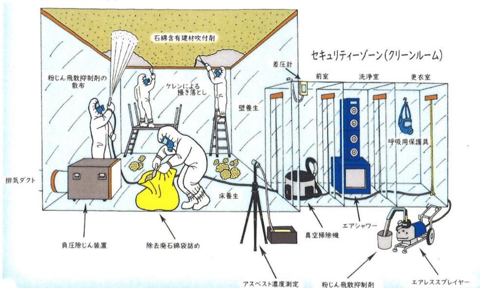
除去作業イメージ図
